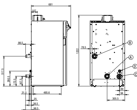
Attacchi idraulici Power HT+ 1.130-1.150
