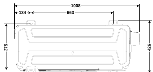
Dima di montaggio
