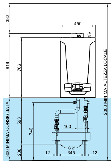
Centrale termica con separatore idraulico
