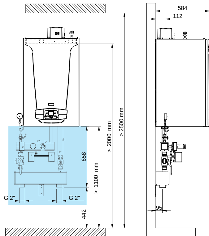
Centrale termica con separatore idraulico
