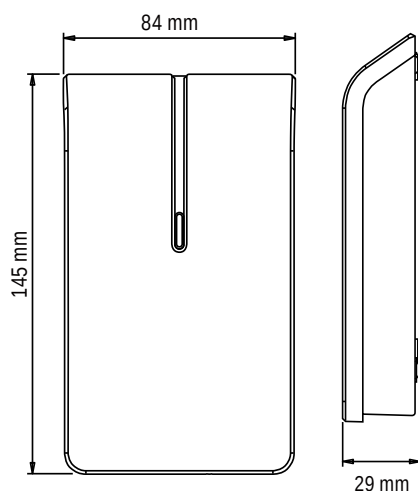
KIT ADATTATORE (GATEWAY) BAXI MAGO
