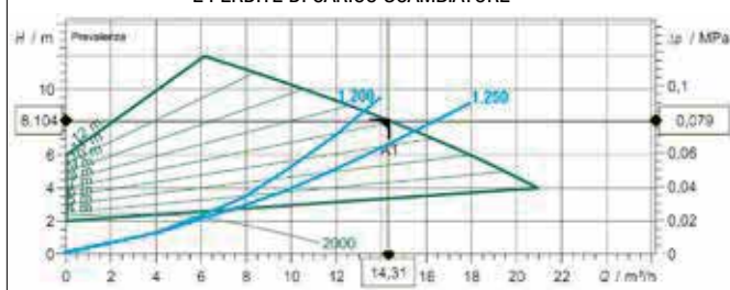
CURVA CARATTERISTICA CIRCOLATORE POWER HT+ 1.200-1.250 E PERDITE DI CARICO SCAMBIATORE
