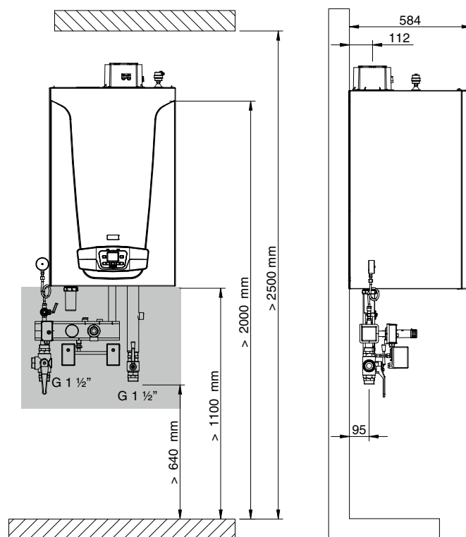
Centrale termica con scambiatore a piastre
