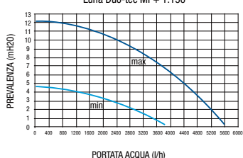
CURVA PORTATA PREVALENZA POMPA ALLA PLACCA Luna Duo-tec MP+ 1.150
