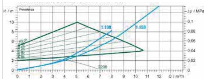
CURVA CARATTERISTICA CIRCOLATORE POWER HT+ 1.130 - 1.150 E PERDITE DI CARICO SCAMBIATORE
