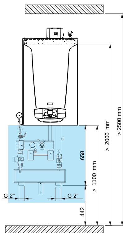
Centrale termica con separatore idraulico
