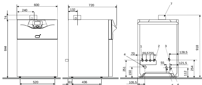
Power 1.32 Solo riscaldamento
