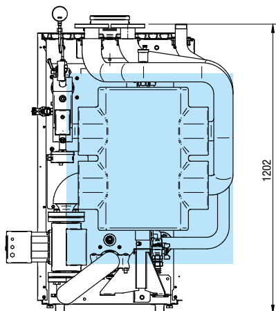
Centrale termica con separatore idraulico
