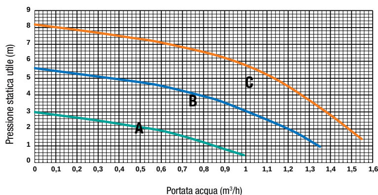
Pompa di circolazione principale
