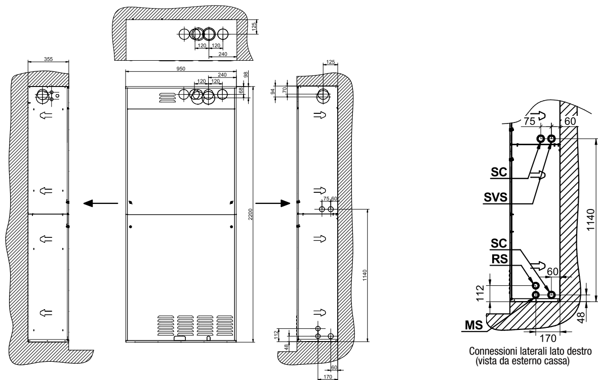
Dima di montaggio
