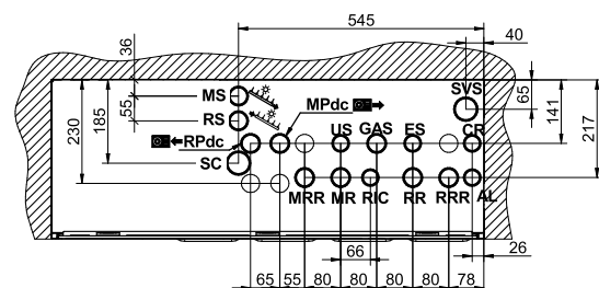
Conessioni fondo cassa (vista da interno cassa)
