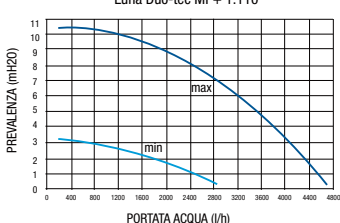
CURVA PORTATA PREVALENZA POMPA ALLA PLACCA Luna Duo-tec MP+ 1.110
