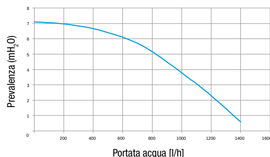
Pompa kit zona miscelata
