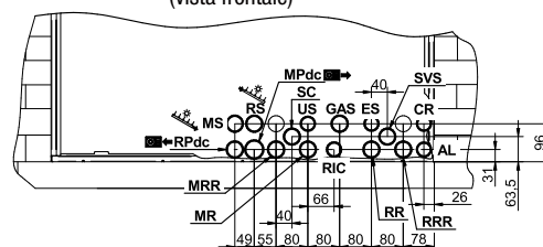
Installazione posteriore (vista frontale)
