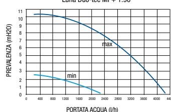
CURVA PORTATA PREVALENZA POMPA ALLA PLACCA Luna Duo-tec MP+ 1.90
