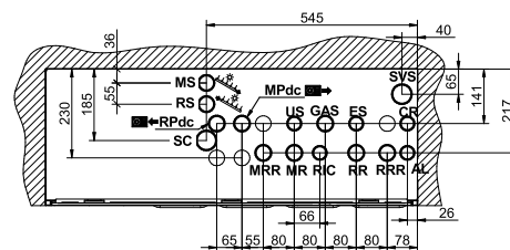
Connessioni fondo cassa (vista da interno cassa)
