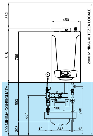
Centrale termica con separatore idraulico
