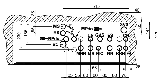
Connessioni fondo cassa (vista da interno cassa)
