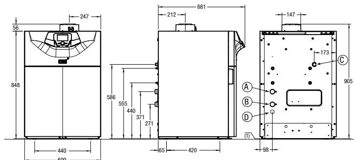
Attacchi idraulici Power HT+ 1.50-1.70
