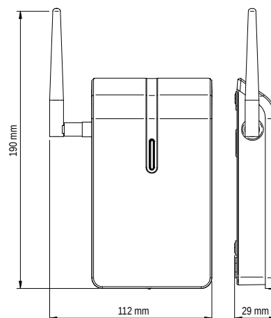
KIT ADATTATORE (GATEWAY) BAXI MAGO WIRELESS
