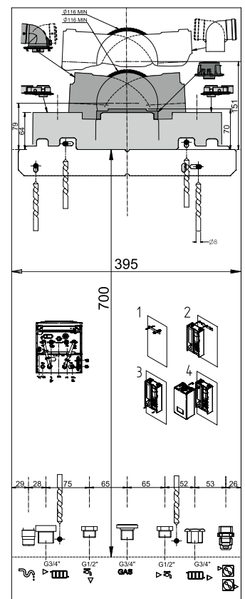
Dima di montaggio
