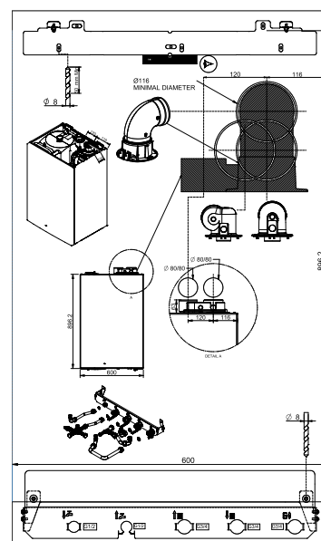
Dima di montaggio
