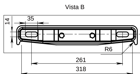
Dimensioni staffa di sostegno
